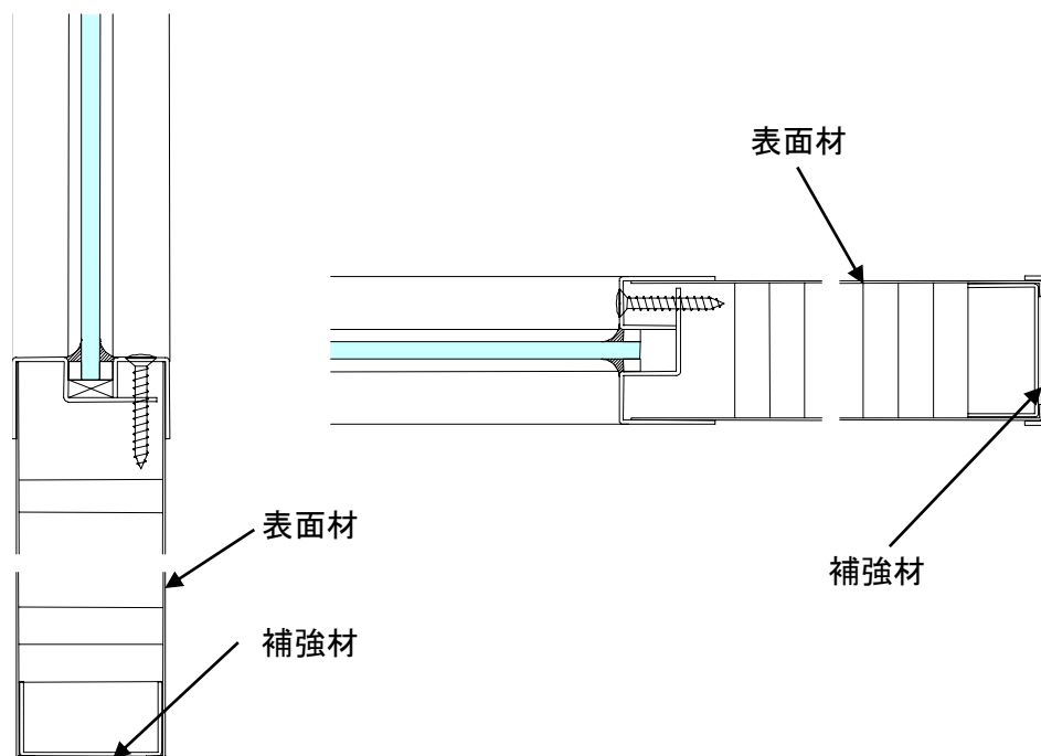
【扉縦断面】
