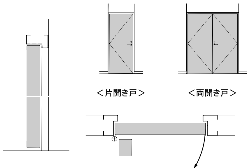
開き式(常時閉鎖方式)
