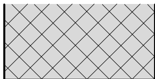
ひし(菱)網入板ガラス
